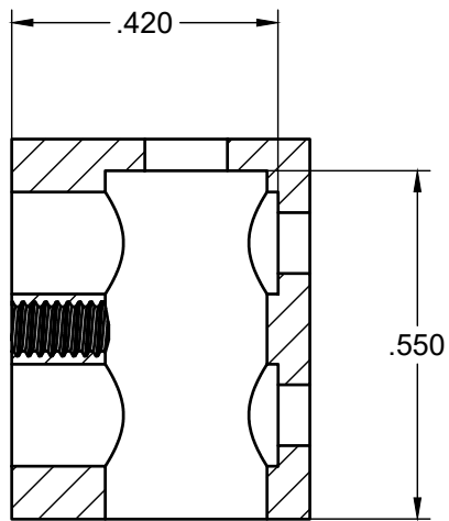
SECTION A-A SCALE 3:1
